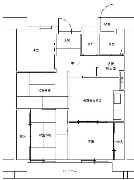
061114 片廊下型 ( 6戸 ) 4DK 浴槽 6.0和, 6.0和, 5.0洋, 5.0洋
