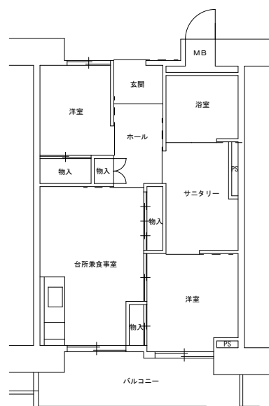
061115 片廊下型 ( 1戸 ) 2DK 浴槽 6.0洋, 4.5洋
