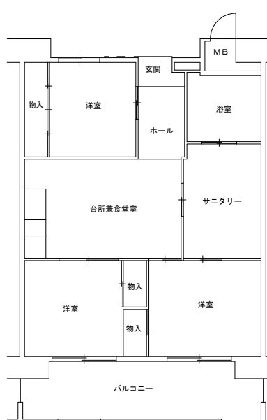
061116 片廊下型 ( 1戸 ) 3DK 浴槽 7.0洋, 6.0洋, 5.0洋
