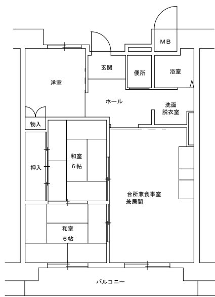
061113 片廊下型 ( 7戸 ) 3LDK 浴槽 6.0和, 6.0和, 5.0洋
