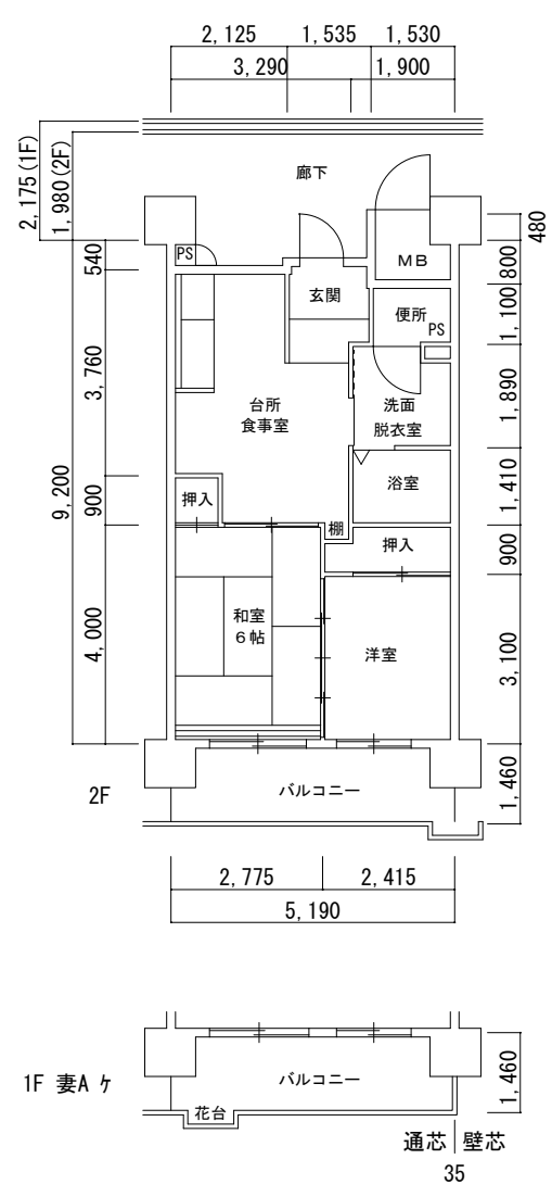
1号館 2DK-A ケ 2DK-A 妻A ケ
