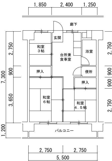
1, 2, 5, 6 号館 3DK
