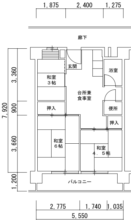
7 号館 3DK
