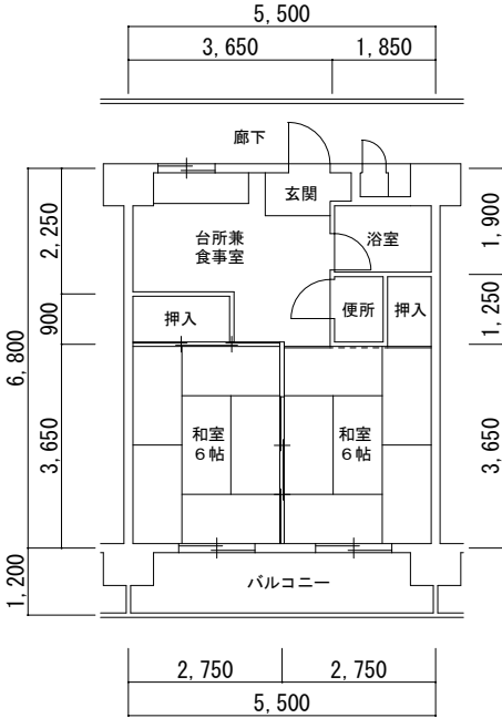
3, 4 号館 2DK
