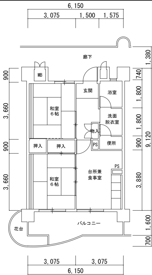
2DK (93108) 41号館
