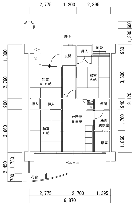
3DK (90107) 41号館
