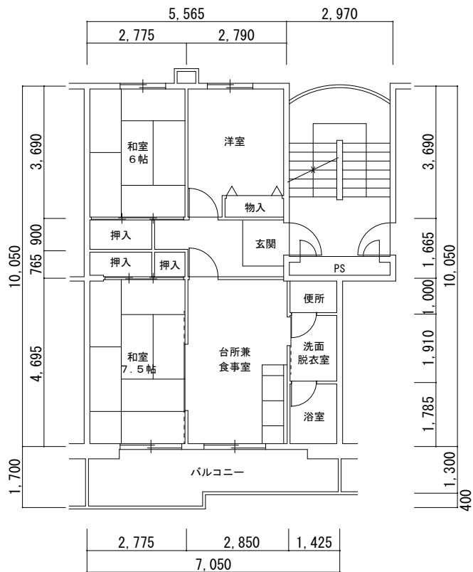
2 4 , 2 5 号 館 ( 8 4 1 0 2 )
