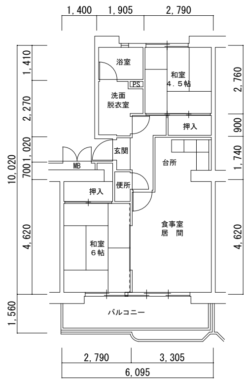
2 6 号 館 ( 8 6 1 1 6 )
