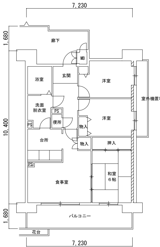
3DK-B 57号館
