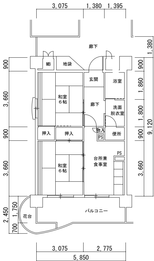
2DK (90108) 41号館
