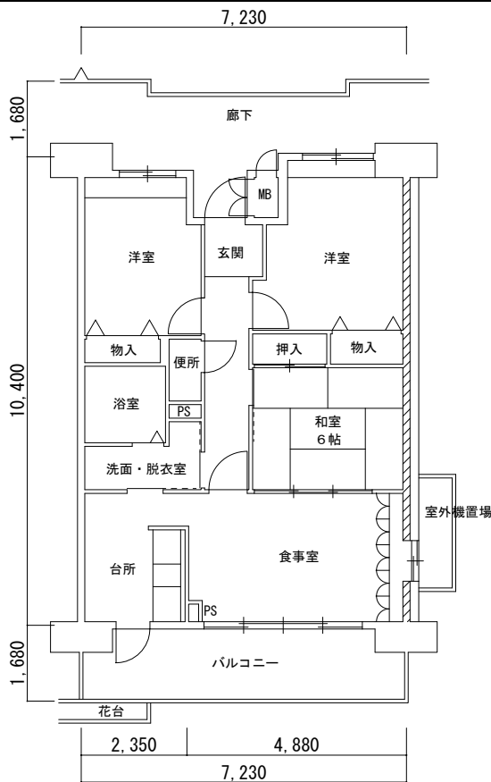
3DK-A 57号館
