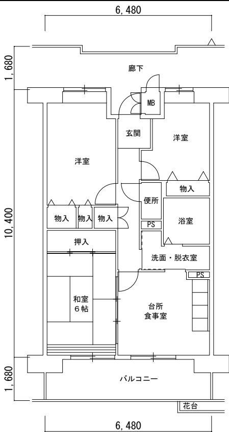
3DK 57号館
