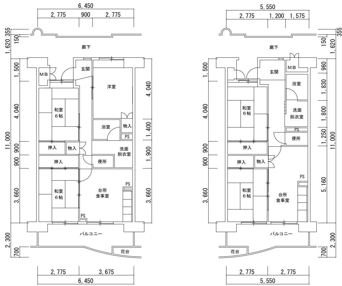
3DK (94102) 51号館
