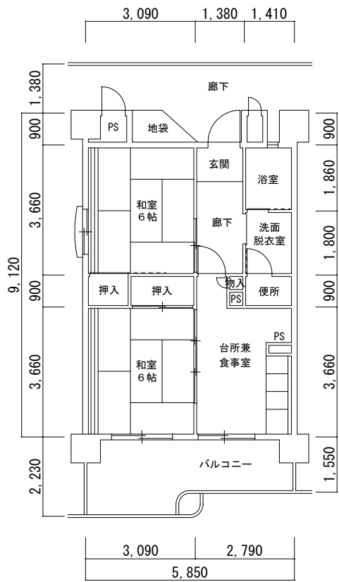
2 4 , 2 5 号 館 ( 8 4 1 0 2 )
