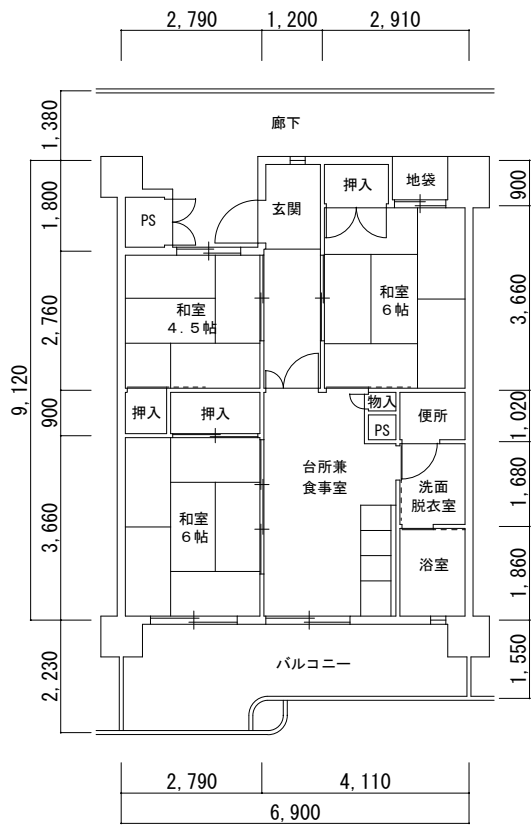
2 4 , 2 5 号 館 ( 8 4 1 0 1 )
