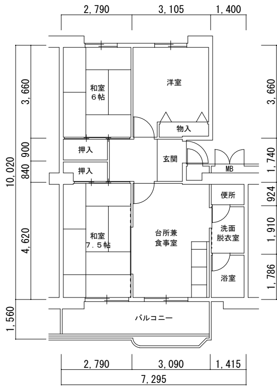
2 6 号 館 ( 8 6 1 0 2 )
