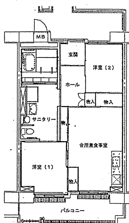
051108 片廊下型 (1戸) 2DK 浴槽 6.0洋,4.5洋
