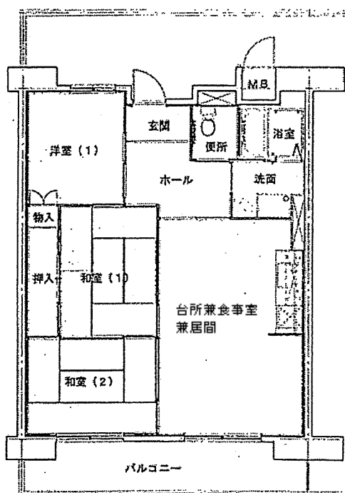
051105 片廊下型 (8戸) 3LDK 浴槽 6.0和,6.0和,5.0洋
