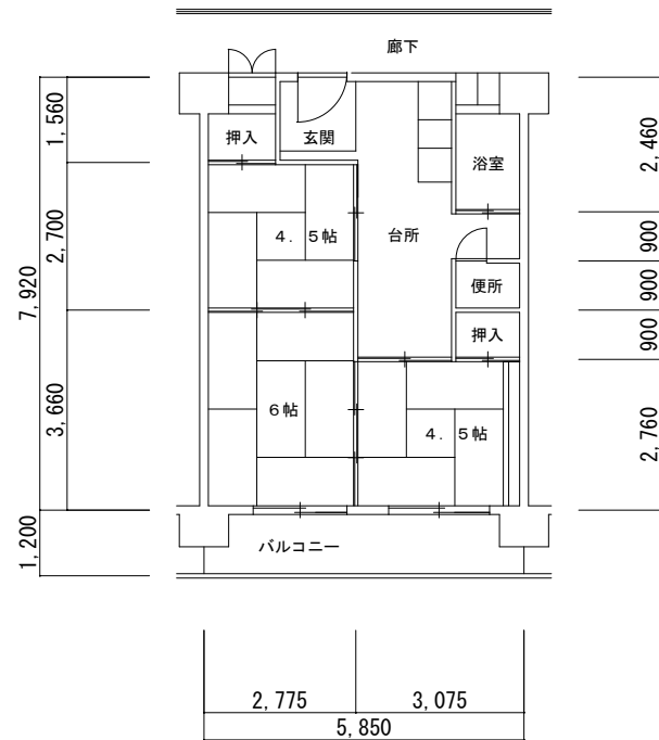
(3DK) 1 号館 (73107-03)
