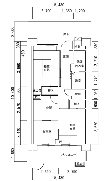
4号館 2DK 老 (96114-06)
