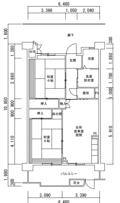
1号館 2LDK-2 (老) (94166-01)
