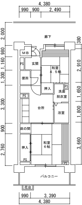
3号館 2K (老) (96169-08)
