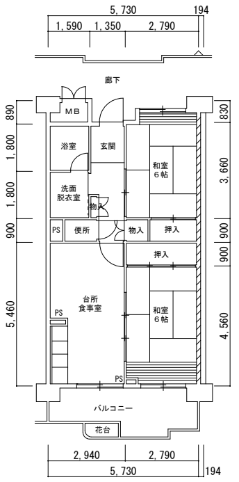
1号館 2DK (94163-01)
