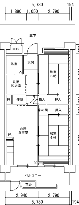
1号館 2DK (老) (94163-02)
