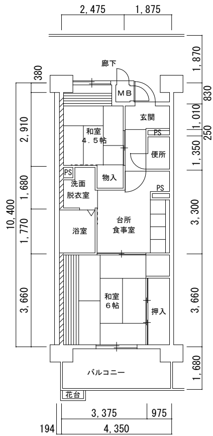
2号館 2K (老)
