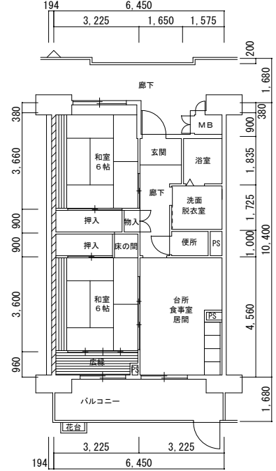
3号館 2LDK (老) (96240-04)
