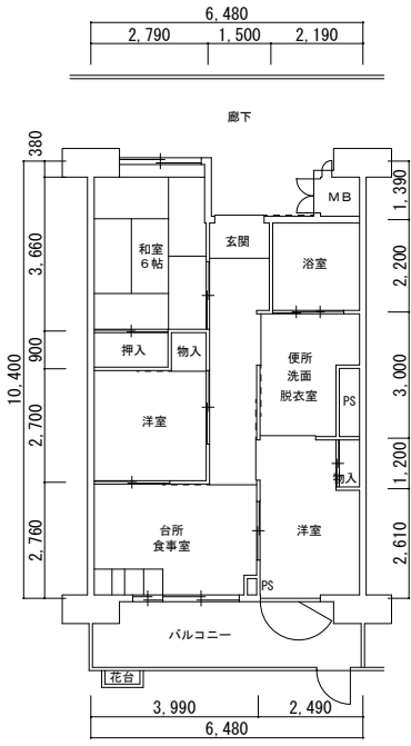
3号館 3DK (身) (96251-01)
