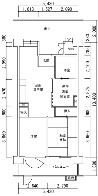
3号館 2DK (身) (96252-01)
