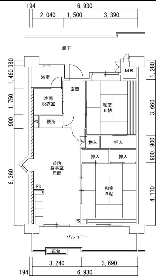
5号館 2LDK (94160-01)
