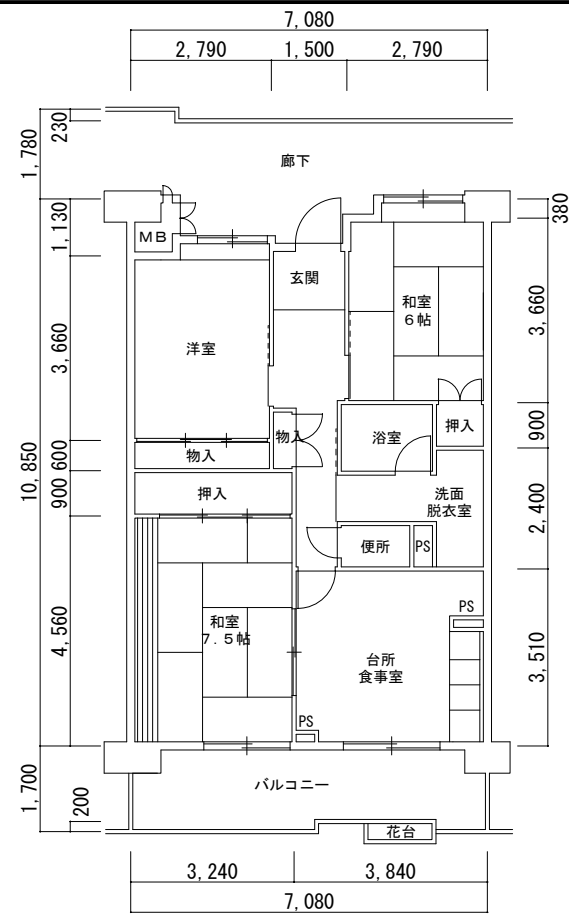
5号館 3DK (94158-01)
