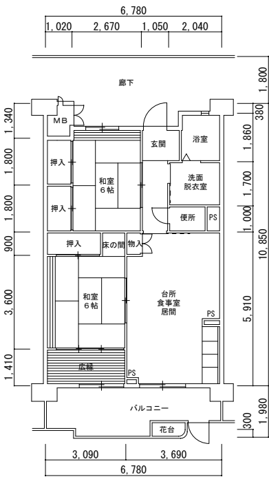
1号館 2LDK (老) (94165-01)
