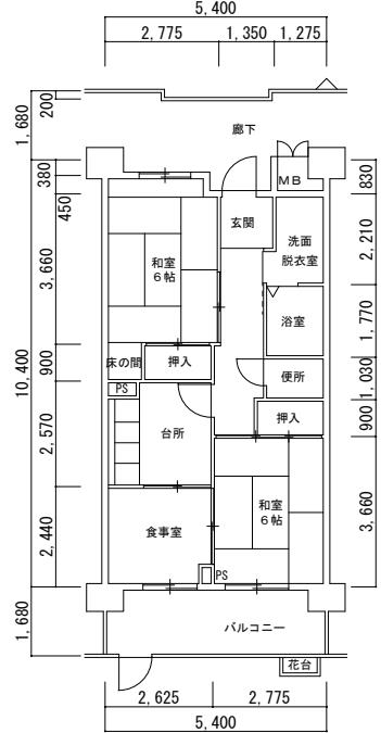
3号館 2DK (老) (96212-05)
