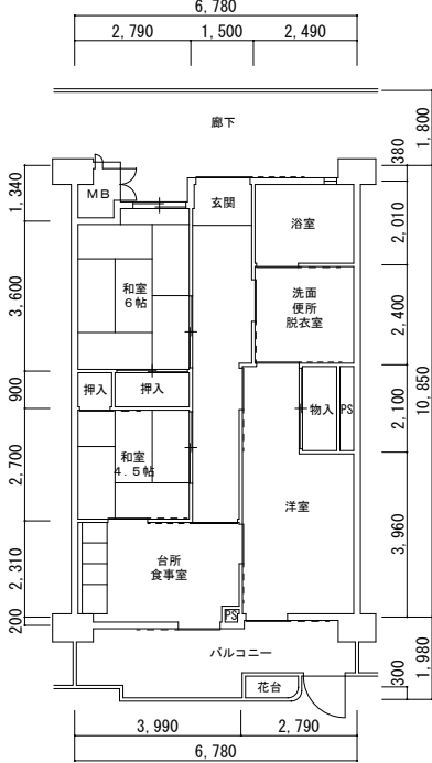
1号館 3DK (身) (94164-02)
