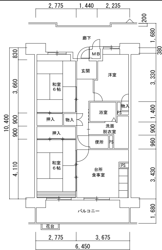
2号館 3DK
