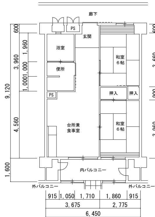
1号館 (77156-01) 2DK 身
