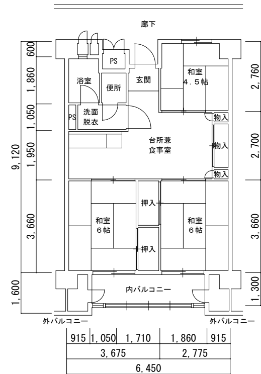
1号館 (77153-02) 3DK
