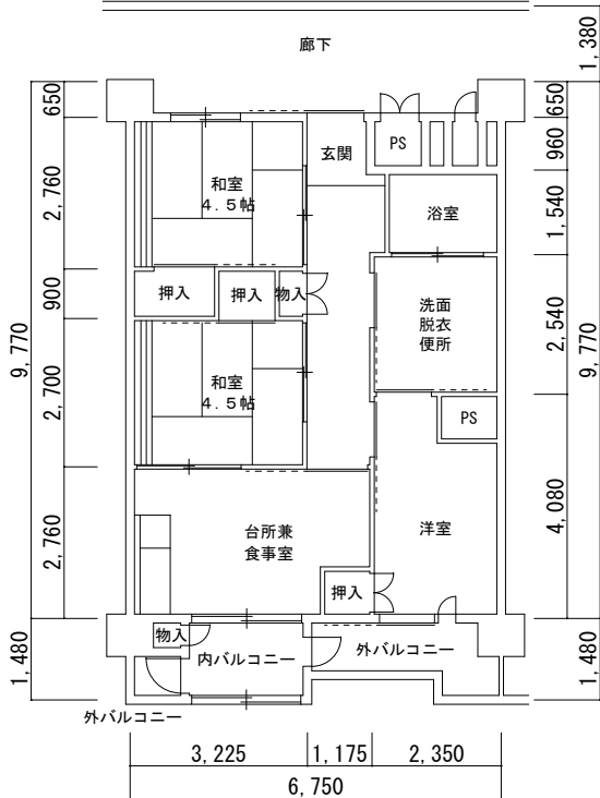
2号館 (85251-01, 02) 3DK 身
