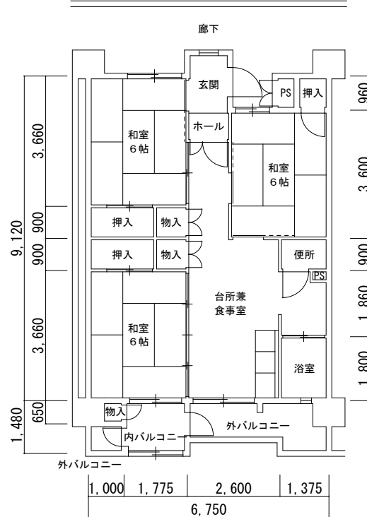
2号館 (85252-01, 02) 3DK
