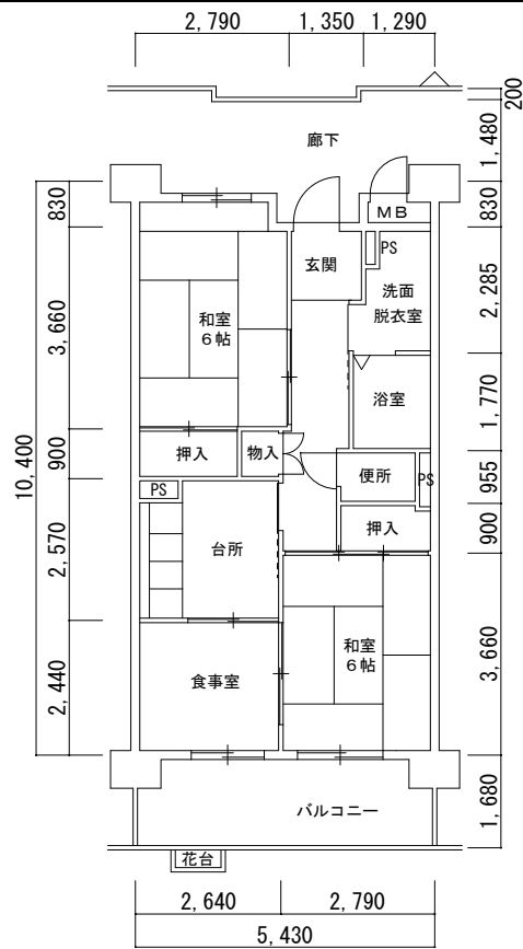
2号館 (02116-02) 2 DK
