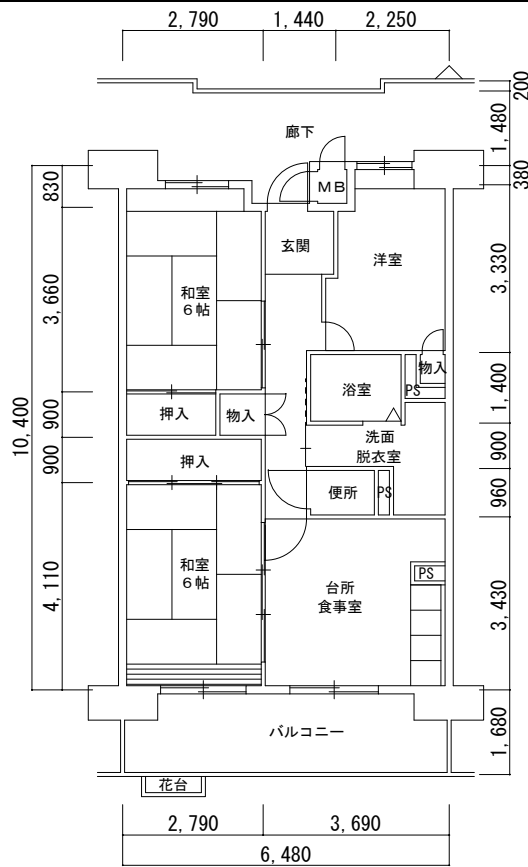
2号館 (02116-03) 3 DK
