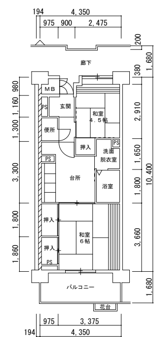
1号館 2K (96180-01)
