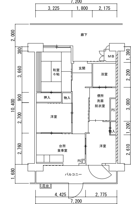
1号館 3DK-2 (96182-01)
