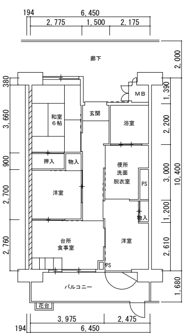
1号館 3DK (96183-01)
