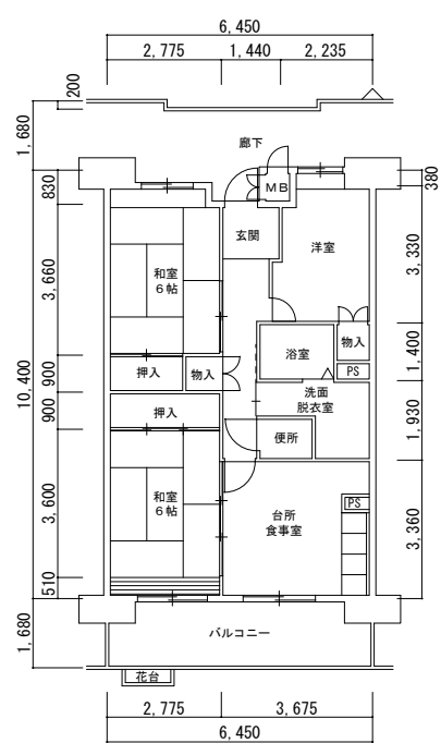
1号館 3DK (96178-01)
