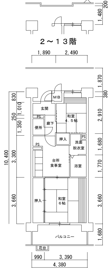
2号館 2K
