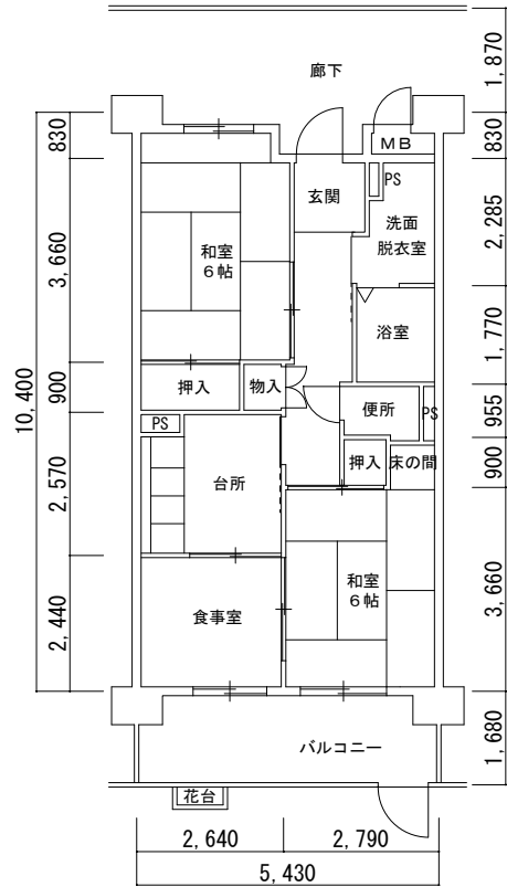
2号館 (02116-07) 2 DK 老
