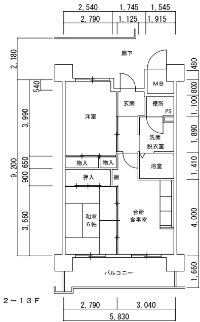
3号館 2DK-B
