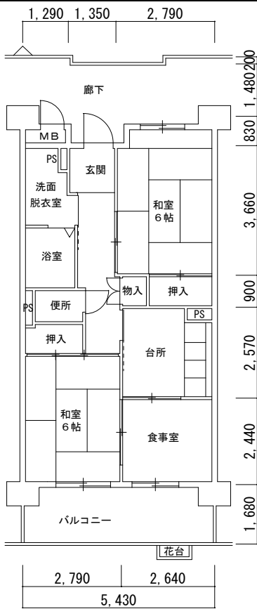
2号館 2DK
