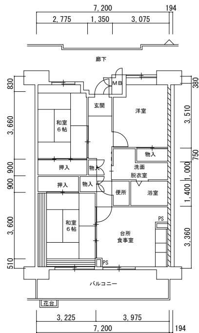
1号館 3DK-2 (96177-01)
