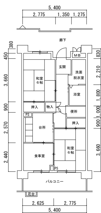
1号館 2DK (96179-01)
