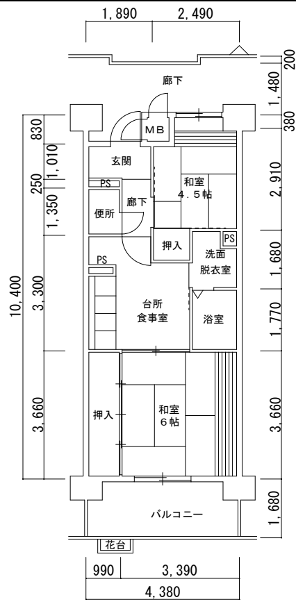
2号館 (02116-01) 2 K
