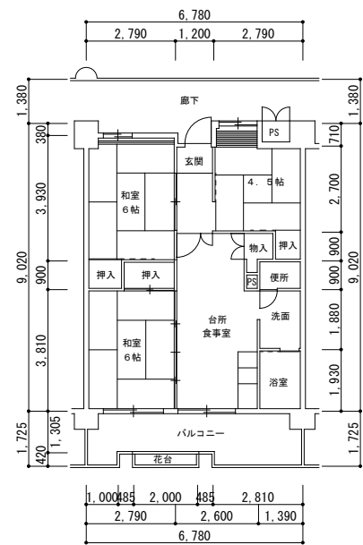
2 号館 3DK (91378-01)
