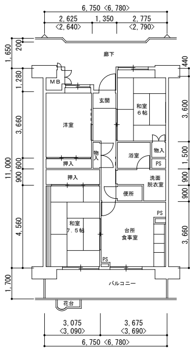
1 号館 3DK (93158-01)
