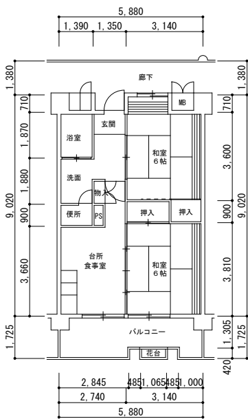
2 号館 2DK (91379-01)
