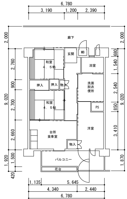
2 号館 3DK (身) (91380-01)
