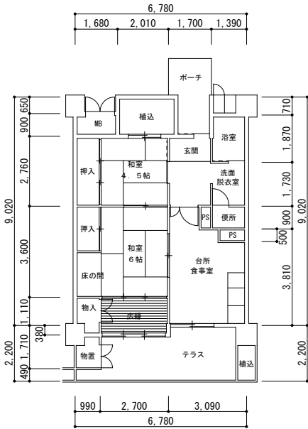
2 号館 2DK (老) (91381-01)
