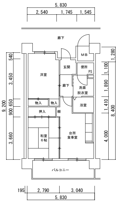
1号館 2DK-B 妻2
