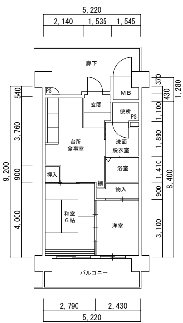
1号館 2DK-A 妻1 (特)
