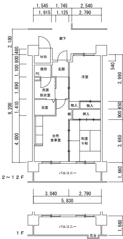
2号館 2DK-B
