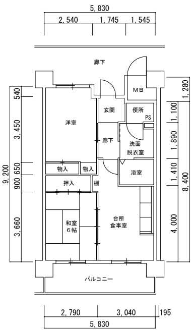
1号館 2DK-B 妻1
