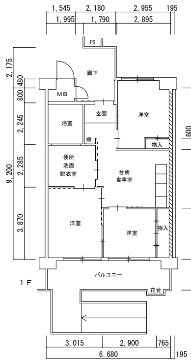
2号館 3DK (妻身)
