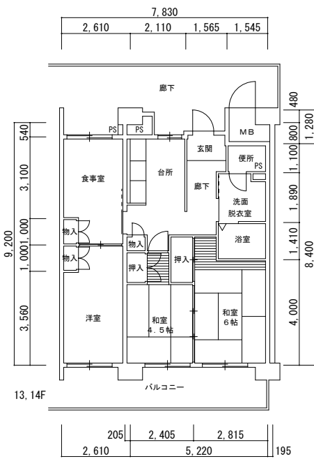
1号館 3DK-2 妻1 (特)
