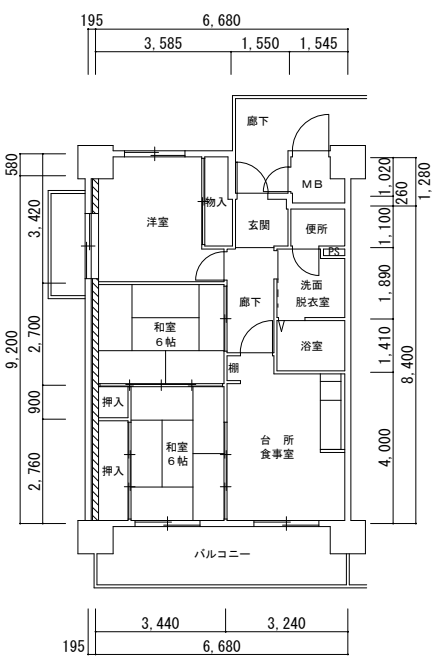
1号館 3DK 妻 (特)
