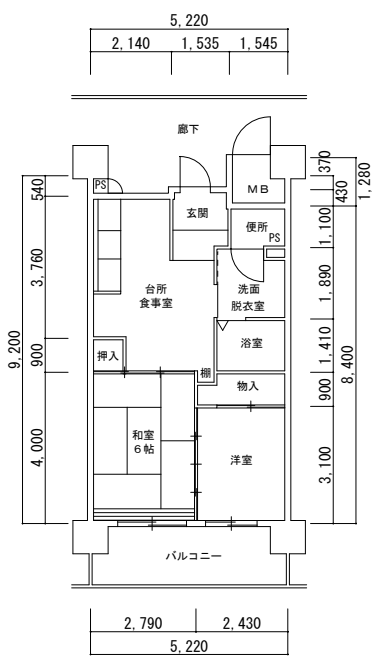
1号館 2DK-A
