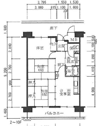
1号館 3DK
