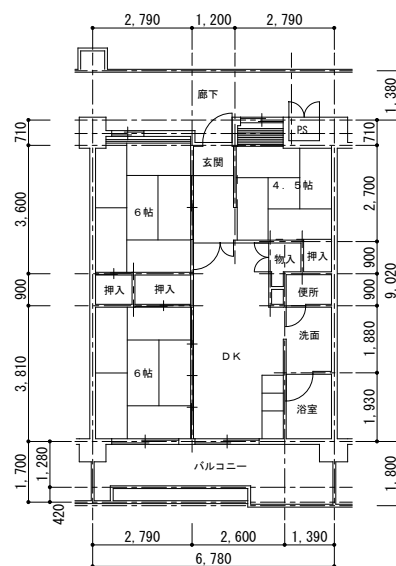
6 号館 (80113)
