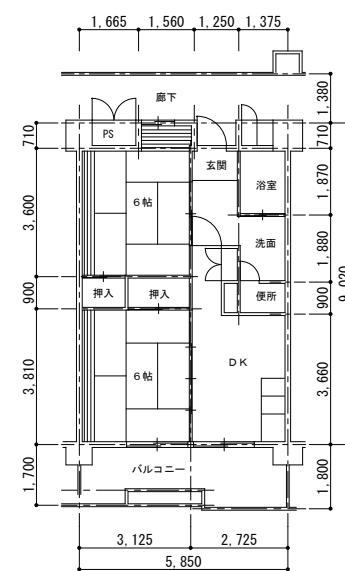
4・5・9 号館 (80119)
