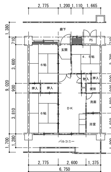
4・5・9 号館 (80120)
