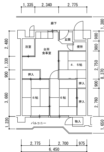
10~12 号館 (身) (77128)
