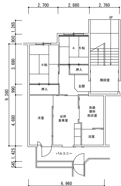
16・17 号館 (身) (84207)
