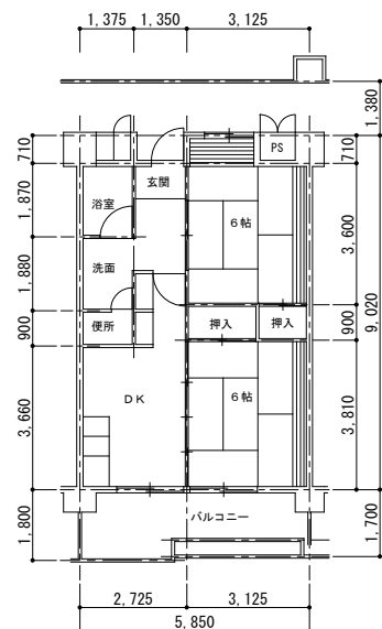
2・3・7・8 号館 (80104)
