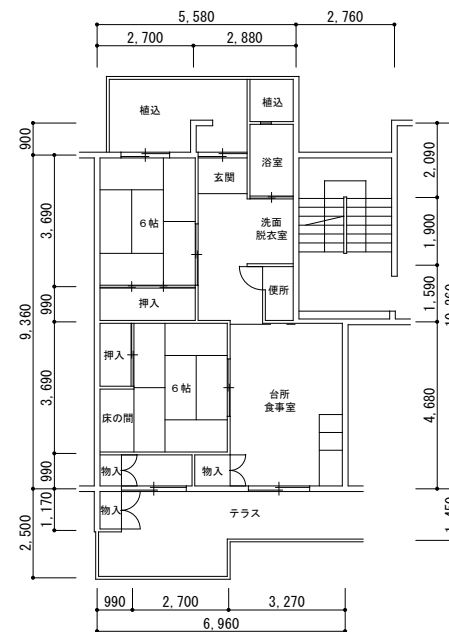
19 号館 (老) (84208)
