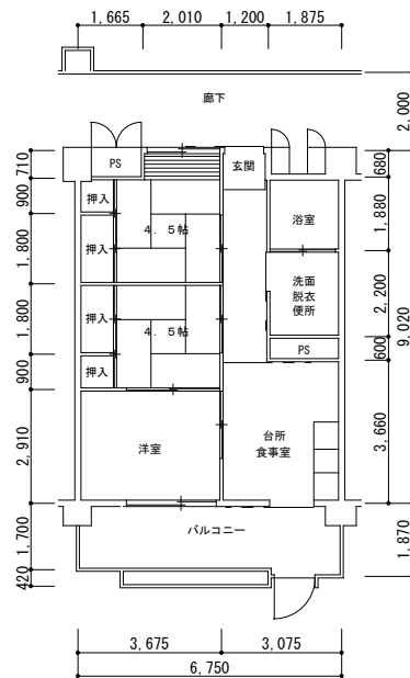
7 号館 (身) (80110)
