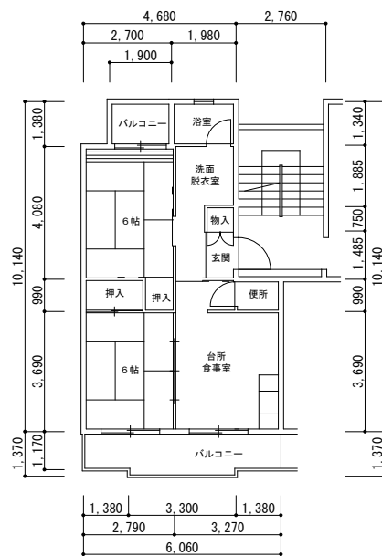
15・17 号館 (身) (84206)
