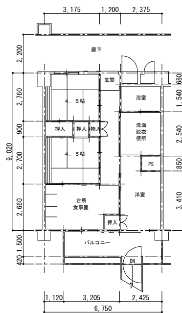
5 号館 (身) (80123)
