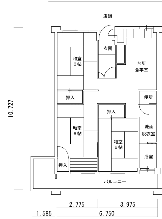
11号館 (86252-01) 3DK
