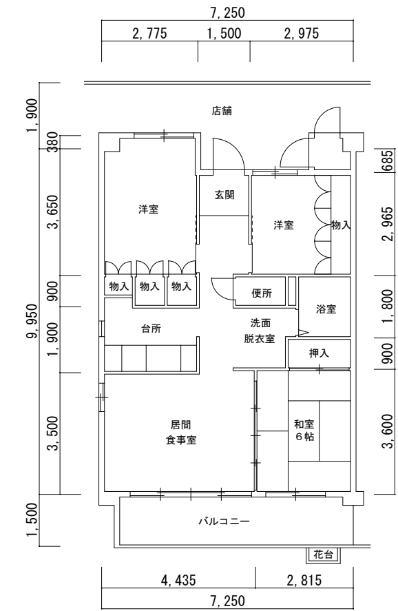
12号館 (00203-01) 3LDK
