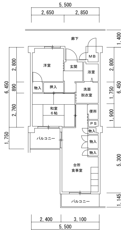
8 号館 (00202-01) (00202-02) 2DK
