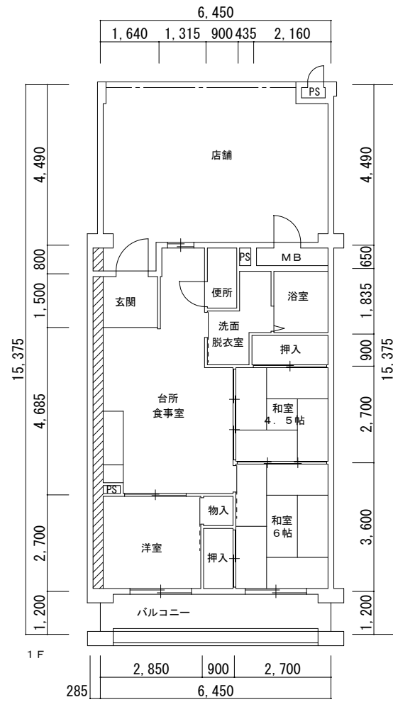
10号館 3DK 店
