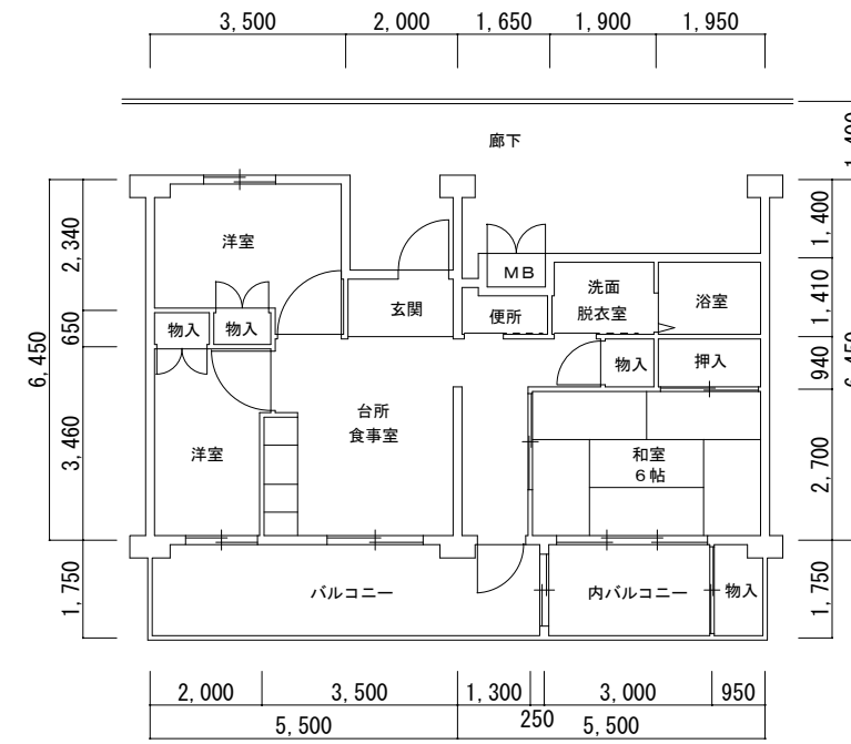
8 号館 (00201-01) 3DK
