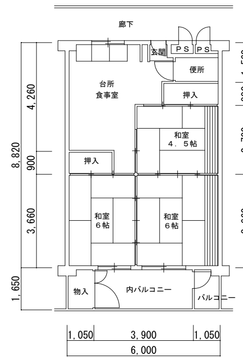
9 号館 (74252-03) 3DK
