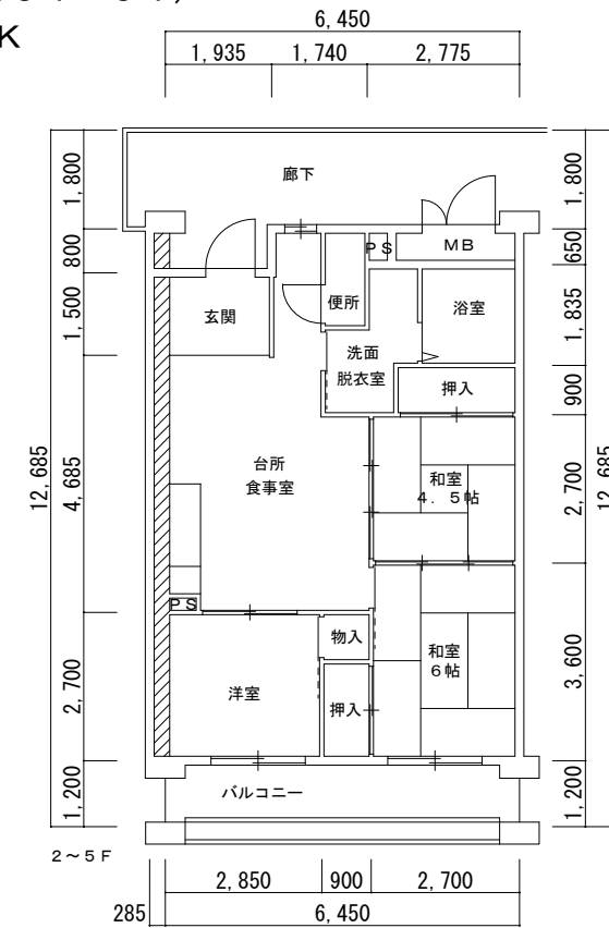
10 号館 3DK
