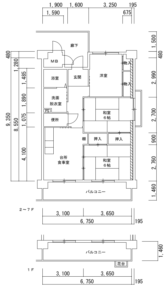
14 号館 3DK 妻
