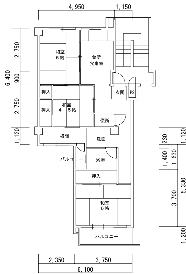
6 号館 (89201-01) 3DK
