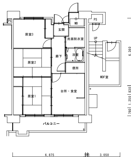
3DK (妻1)
