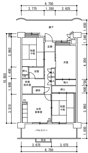
12 号館 3DK 1007 107
