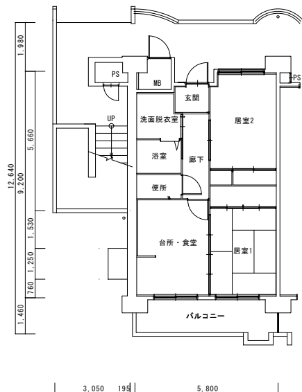
2DK-B (妻1)
