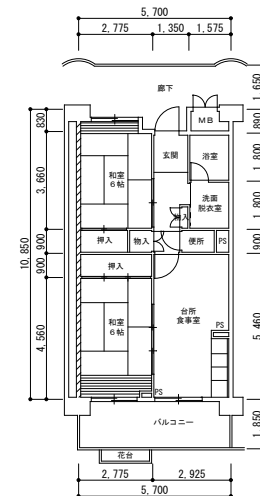
12 号館 2DK 1009 109
