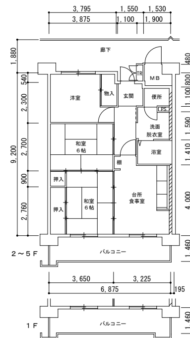
3DK妻
