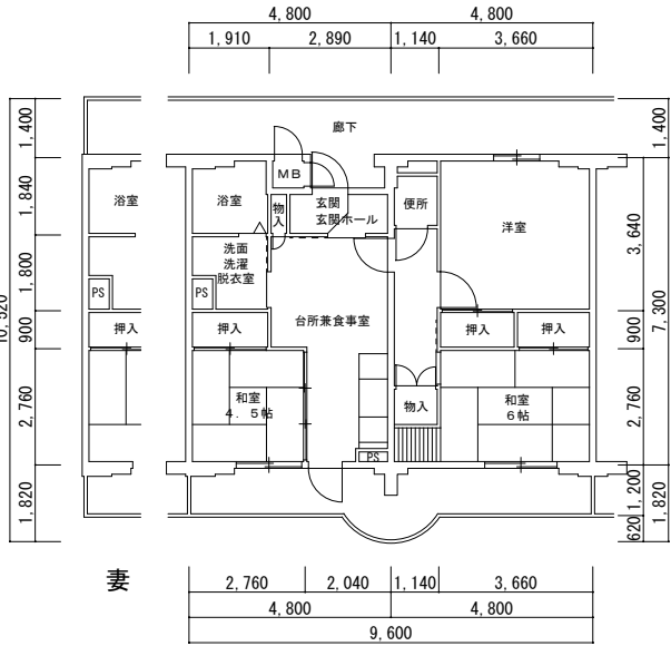
3DK・Aタイプ 9号館（1期） 西棟
