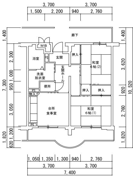
2DK・Bタイプ 9号館（2期） 東棟
