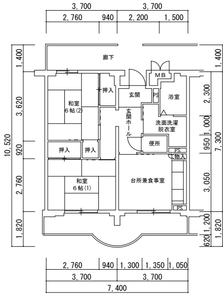
2DK・Bタイプ 9号館（1期） 西棟
