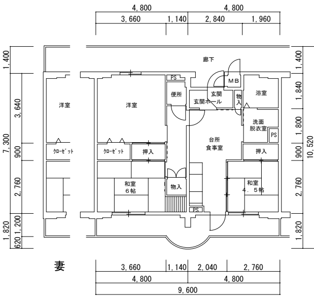
3DK・Aタイプ 9号館（2期） 東棟
