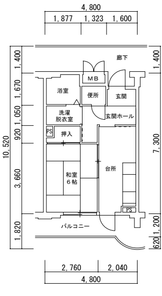
1K 9号館（1期） 西棟
