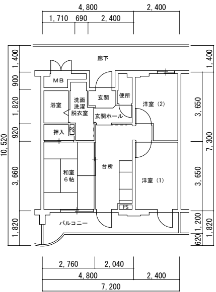
3K・Dタイプ 9号館（1期） 西棟
