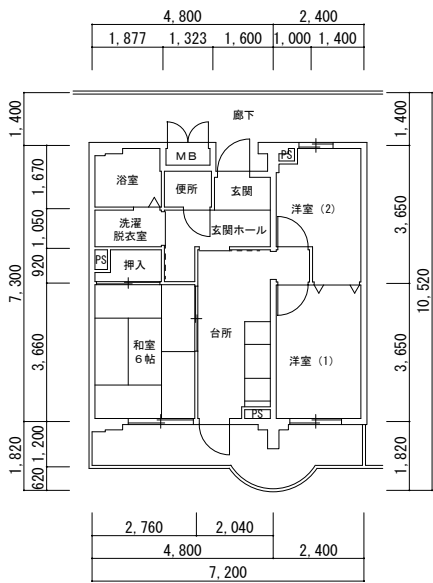
3K・Cタイプ 9号館（2期） 東棟
