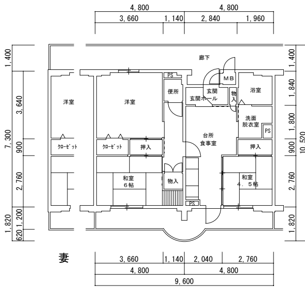
3DK・Bタイプ 9号館（2期） 東棟
