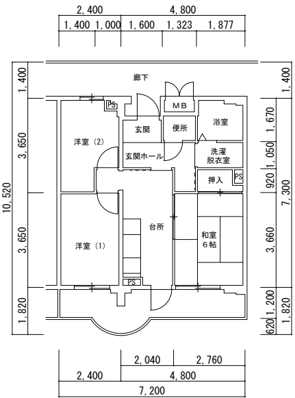
3K・Cタイプ 9号館（1期） 西棟
