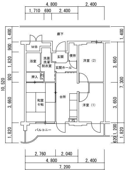
3K・Bタイプ 9号館（1期） 西棟
