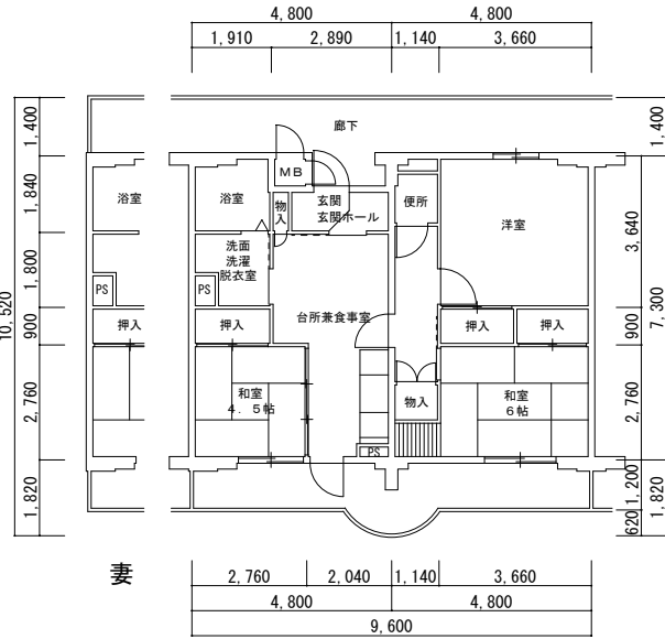
3DK・Bタイプ 9号館（1期） 西棟
