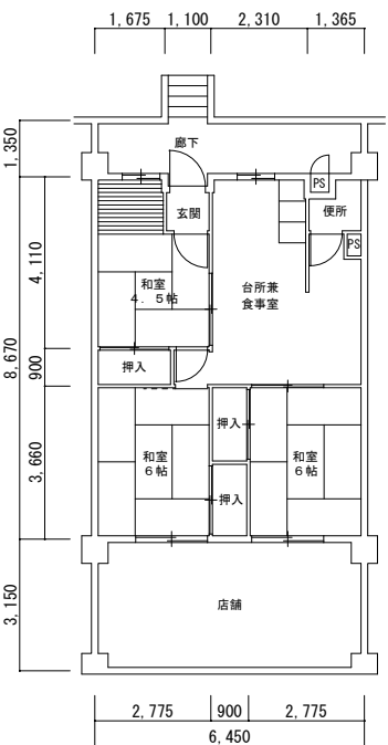
1 2 号館 (76256-03) 3DK店 101・102
