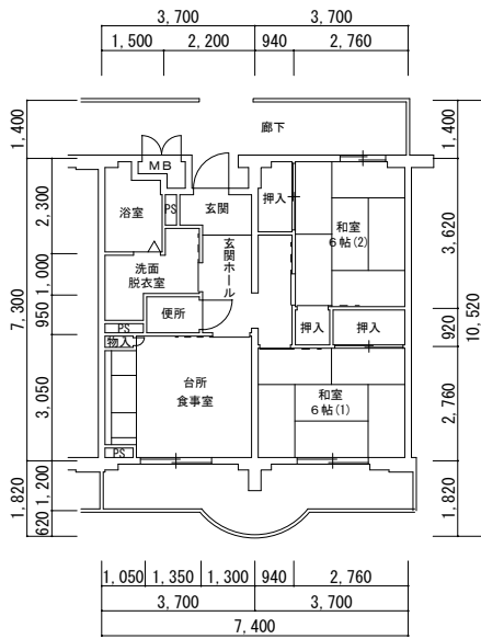
2DK・Aタイプ 9号館（2期） 東棟
