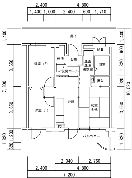
3K・Bタイプ 9号館（2期） 東棟
