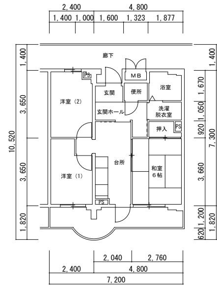
3K・Aタイプ 9号館（1期） 西棟
