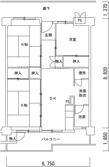
(3DK) 1号館 (80111-03)
