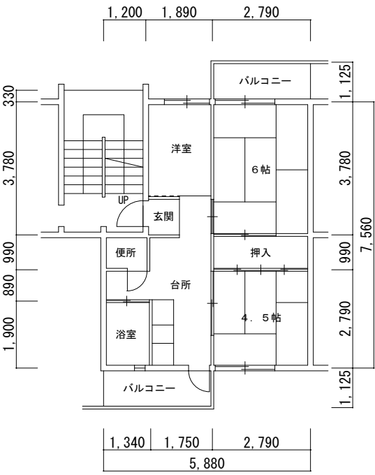
(2DK) 1号館 (80103-02)
