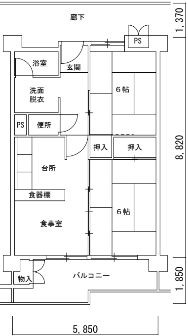
(2DK) 1号館 (80103-02)
