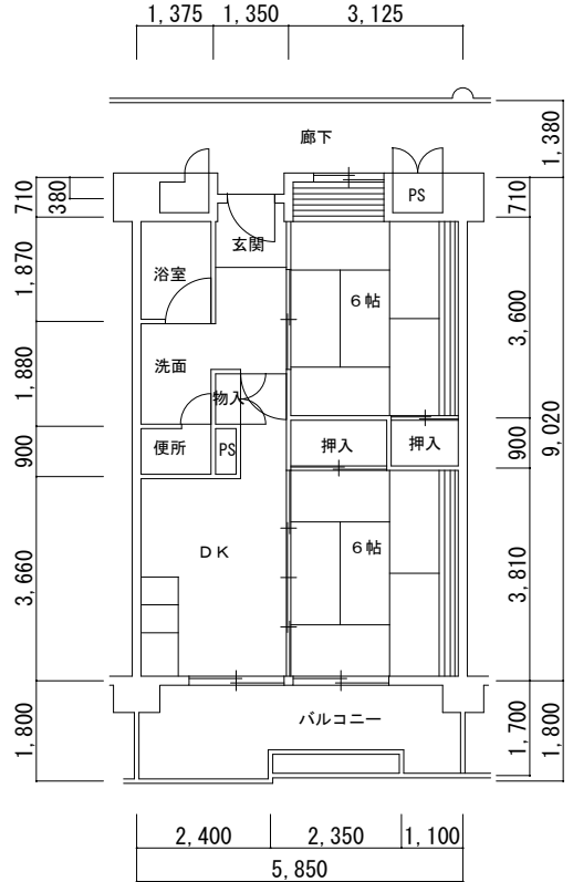
(2DK) 2,3号館 (80105-01,-02)
