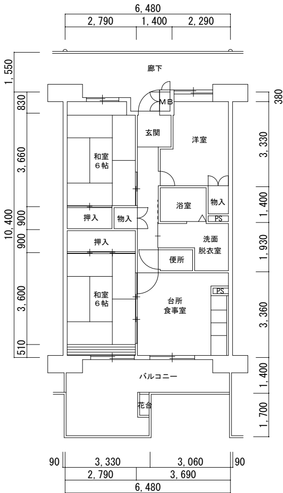
3DK c
