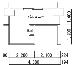
10号館 2K-c
