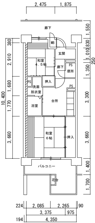
9号館 (02022-06) 2K-a
