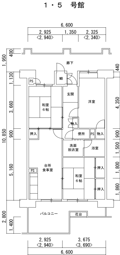
3DK-1 (94147)
