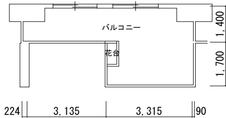
3DK b
