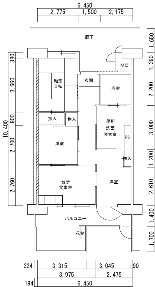
3DK 身 a
