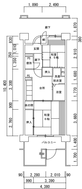
10号館 2K 老
