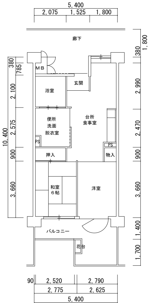
2DK 身
