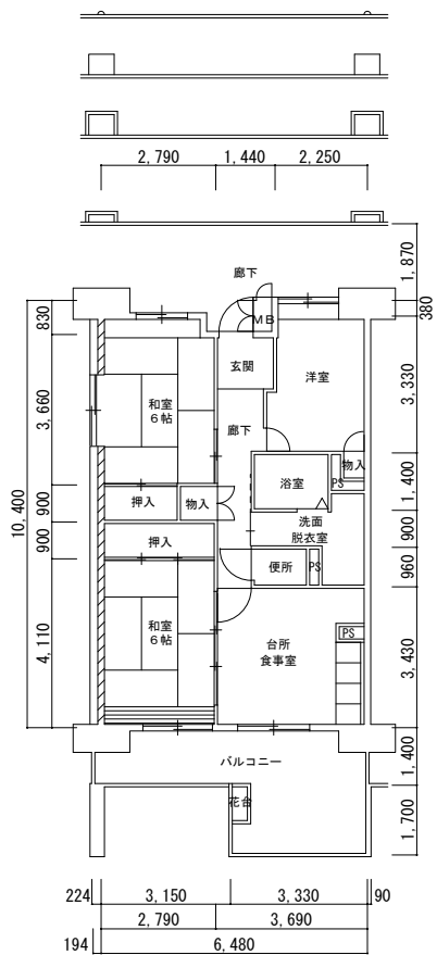
10号館 3DK-a
