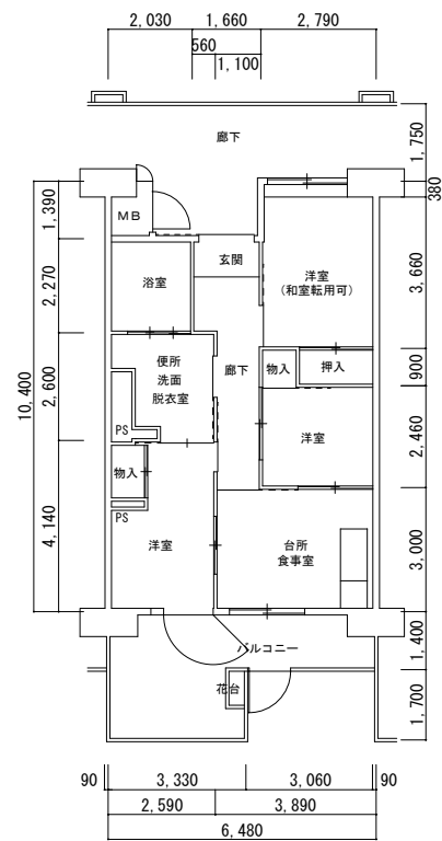
10号館 3DK 身
