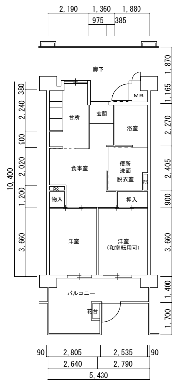
10号館 2DK 身
