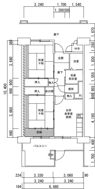
10号館 2LDK 老
