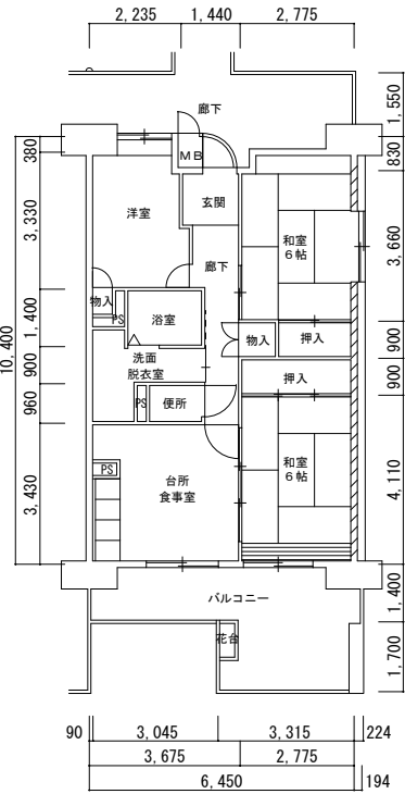
9号館 (02024-05) 3DK-b
