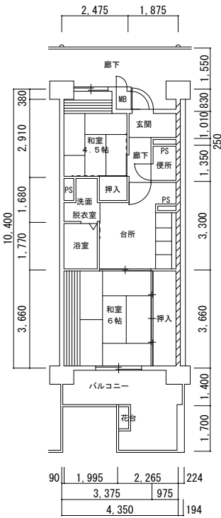
8号館 (02022-04) 2K-d
