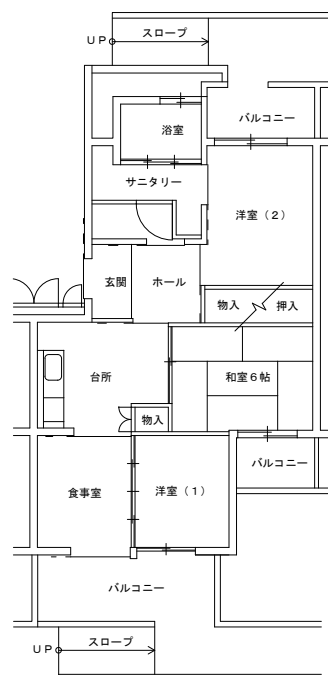
962006 階段室型 ( 2戸 ) 3DK 浴槽 6.0和, 6.0洋, 4.5洋
