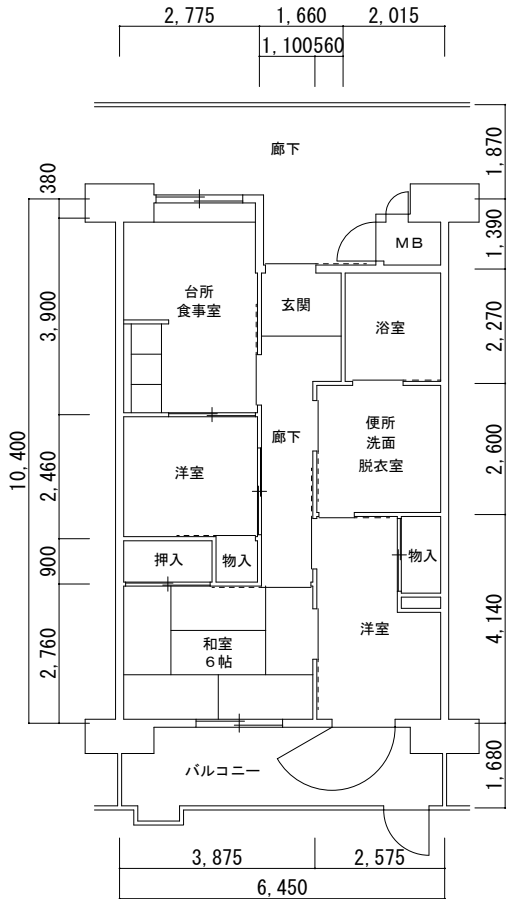
5号館 (02616-01) 3 DK 車
