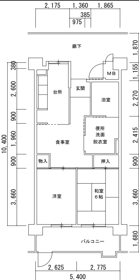
5号館 (02615-01) 2 DK 車
