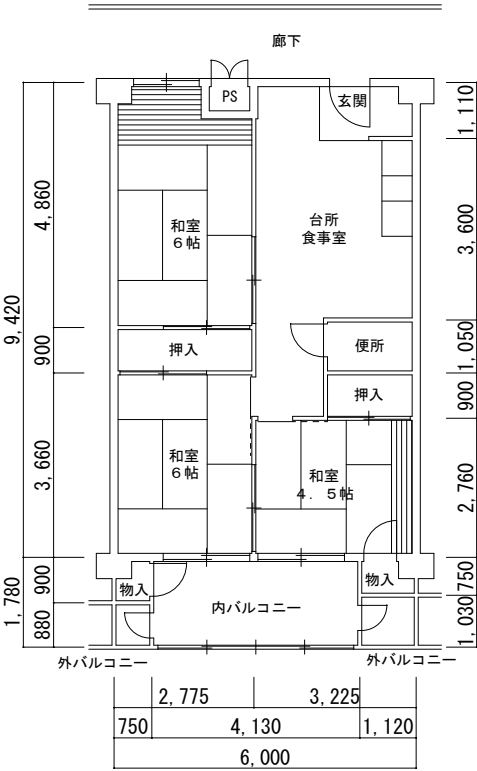
3号館 3DK
