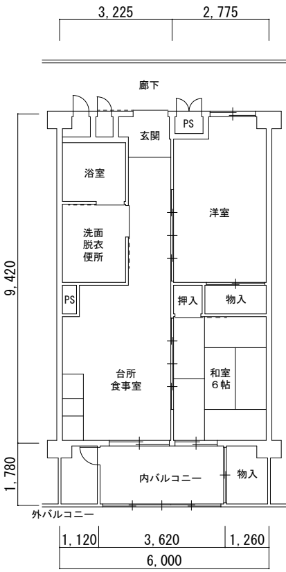
3号館 2DK身
