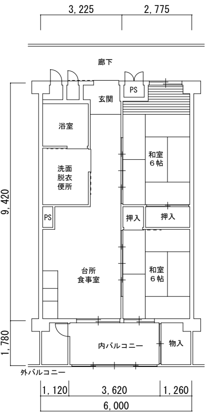
3号館 2DK身
